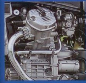
Seziert: › Hondas ganz erstaunlicher CX-500-Motor
