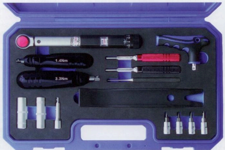
Im Programm: ein 15-teiliger Werkzeugsatz für Reifendruck-Kontrollsysteme.
